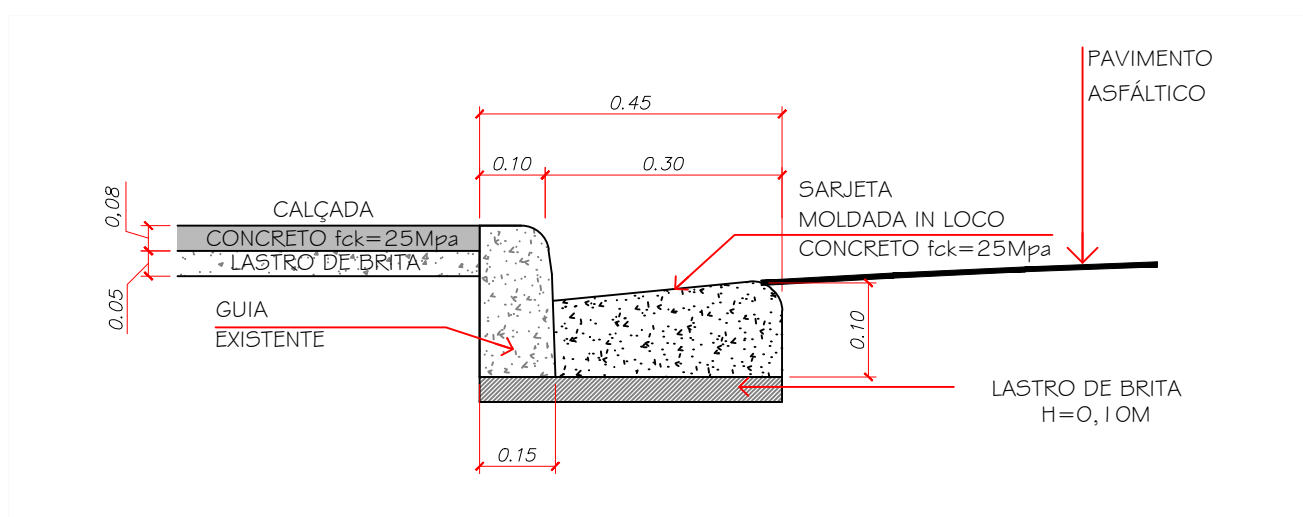
DETALHE GUIA/SARJETA ESCALA 1:15
